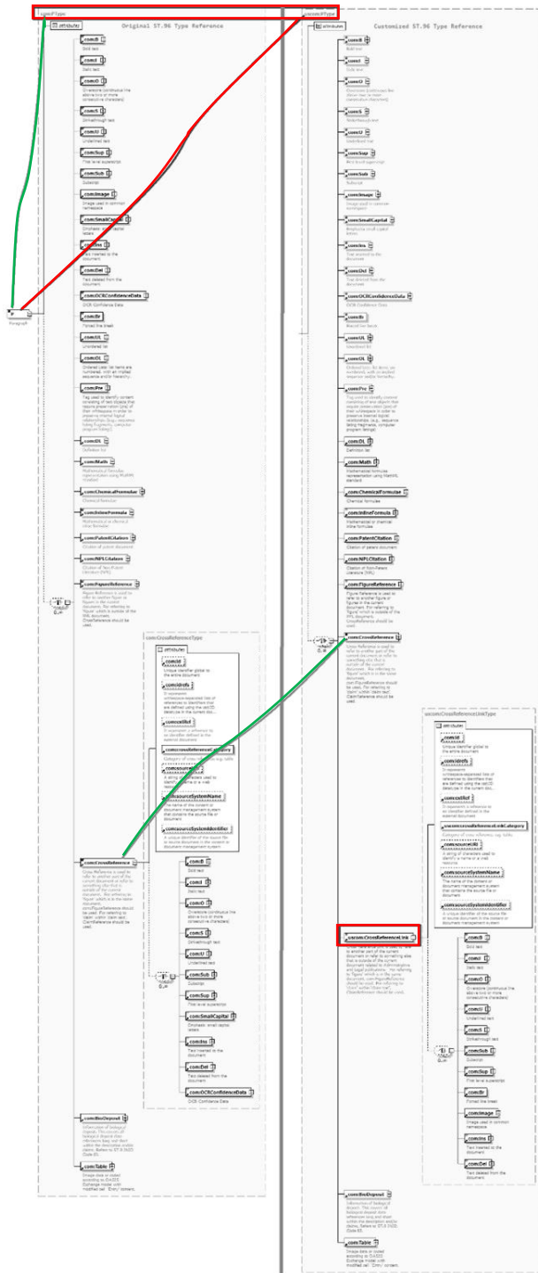
Figura 10: Diagrama del esquema XSD actualizado
